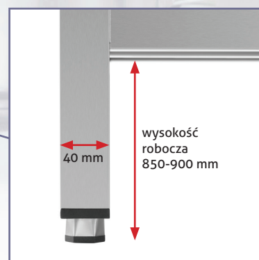
Noga z profilu kwadratowego chromowo-niklowego 1.4301, przekrój 40x40 mm, regulowana -10/+60 mm, łącznie 60 mm. Możliwość zwiększenia wysokości z 850 do 900 mm
