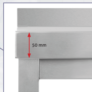
Blat z matowej polerowanej stali chromowo-niklowej 1.4301, narożniki wypawane i wypolerowane.
